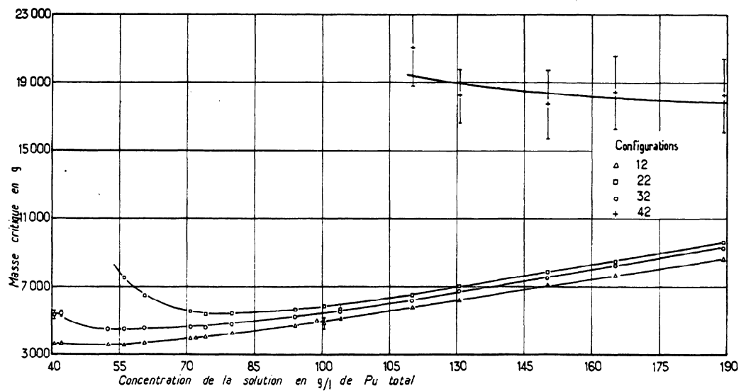
FIG. 5. Cylindre annulaire de 500 mm x 300 mm - Courbes M_c = f(c) pour diverses configurations - Acidité libre 2,1 à 2,4N
