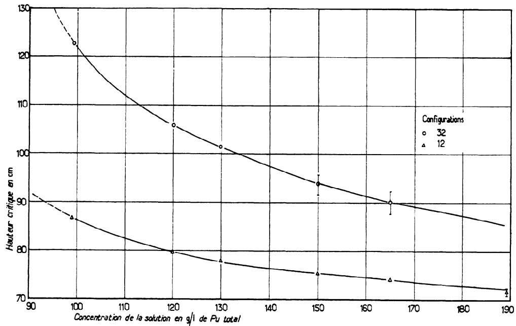
FIG. 18. Cylindre annulaire de 500 mm × 350 mm - Courbes H_c = f(c) pour diverses configurations - Acidité libre 2, 1N
