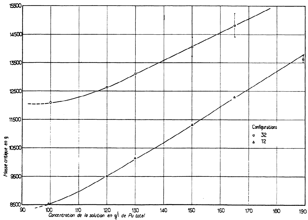
FIG. 19. Cylindre annulaire de 500 mm × 350 mm - Courbes M_c = f(c) pour diverses configurations - Acidité libre 2, 1N
