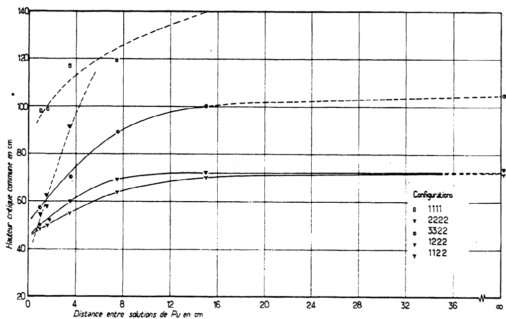
FIG. 9. Interaction entre deux cylindres annulaires de 500 mm x 300 mm pour diverses configurations - Courbes H_C = f(d) - C_{Pu} = 40,6 g/l - Acidité libre 2,2N
