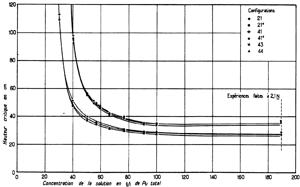
FIG. 13. Cylindre annulaire de 500 mm x 200 mm - Courbes H_c = f(c) pour diverses configurations - Acidité libre 1,6N
